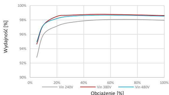
Krzywa wydajności
