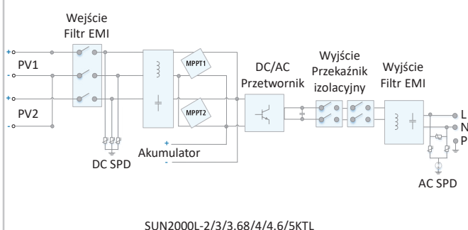
Schemat obwodu
